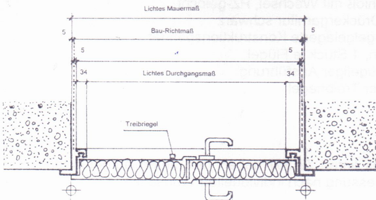
Darstellung Gehfügel DIN rechts
