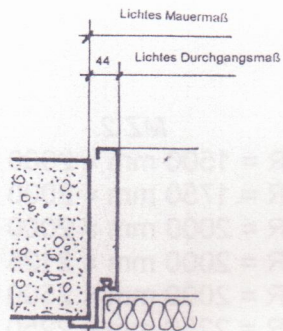
Umfassungszarge
