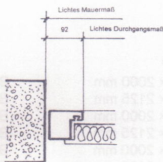
Blockzarge für stumpfen Einbau
