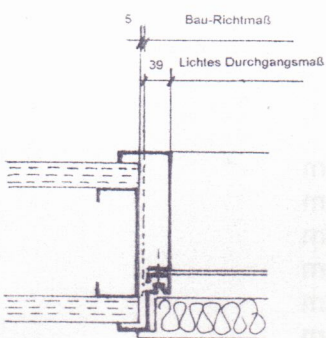
Gegenzarge für Gasbeton- bzw. Ständerwand
