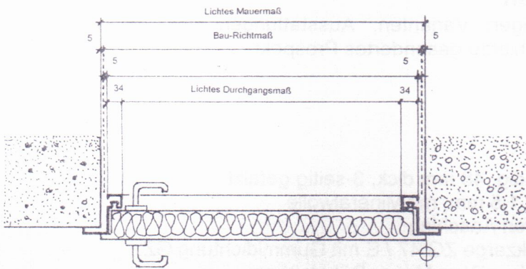
Darstellung DIN rechts
